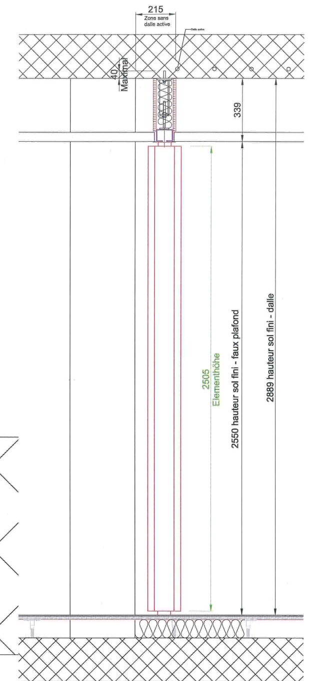
Coupe A-A ( 1:10 )
