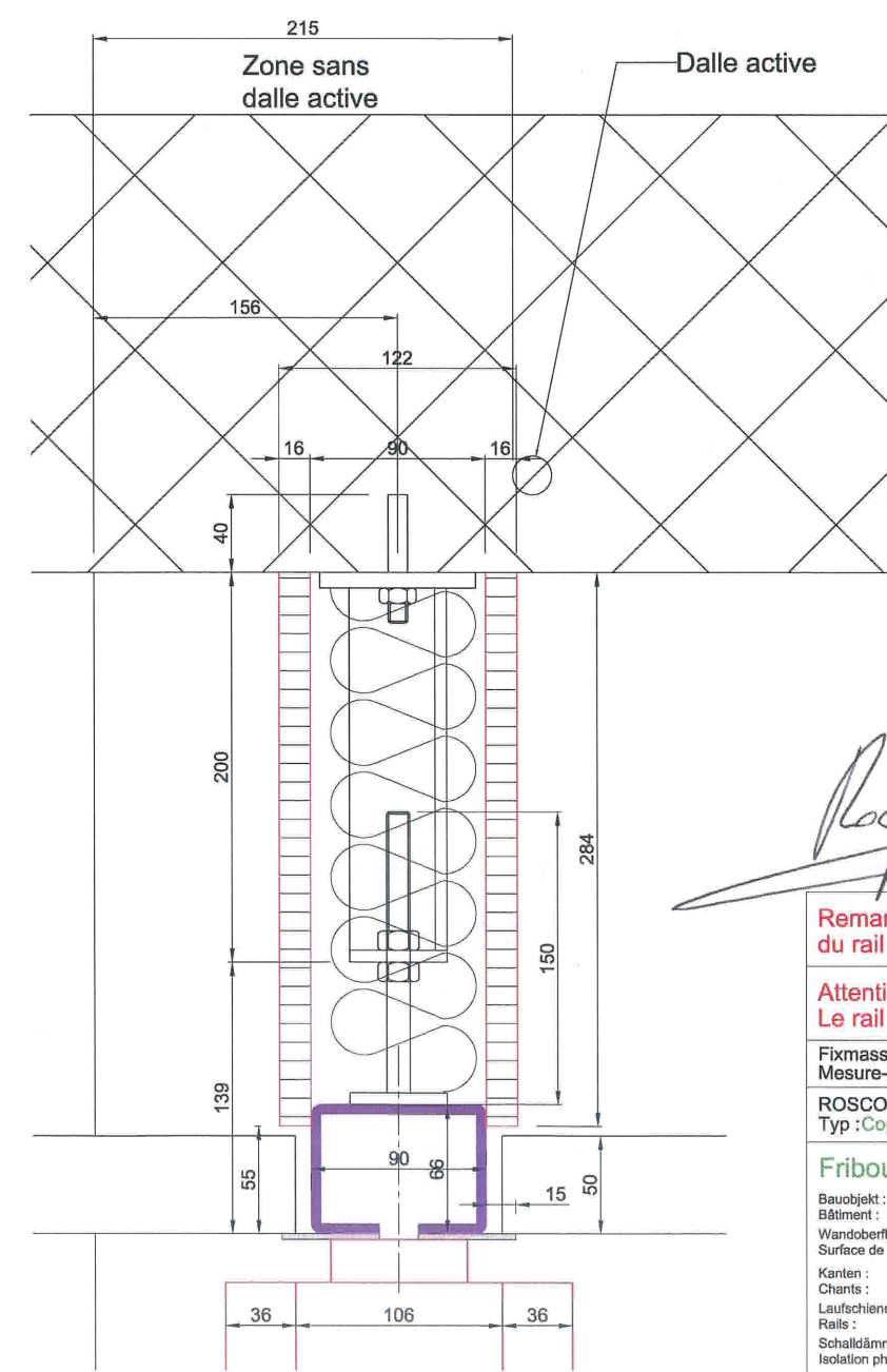
Coupe A-A ( 1:10 )
